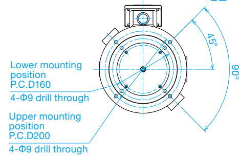
150 L Type
