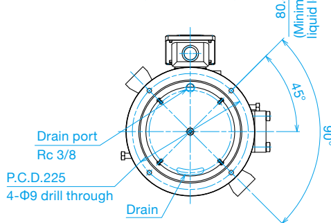
300 L Type
