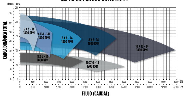
Curva de Familia Serie HC 14"
